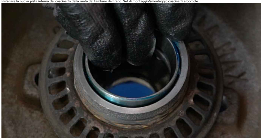
19 Installare la nuova pista interna del cuscinetto della ruota dal tamburo del freno. Set di montaggio/smontaggio cuscinetti e boccole.
