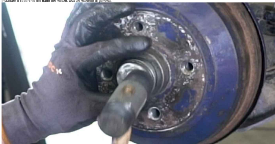
35 Trattare la superficie in cui il cerchio viene a contatto con il freno a tamburo. Utilizzare grasso ceramico.
