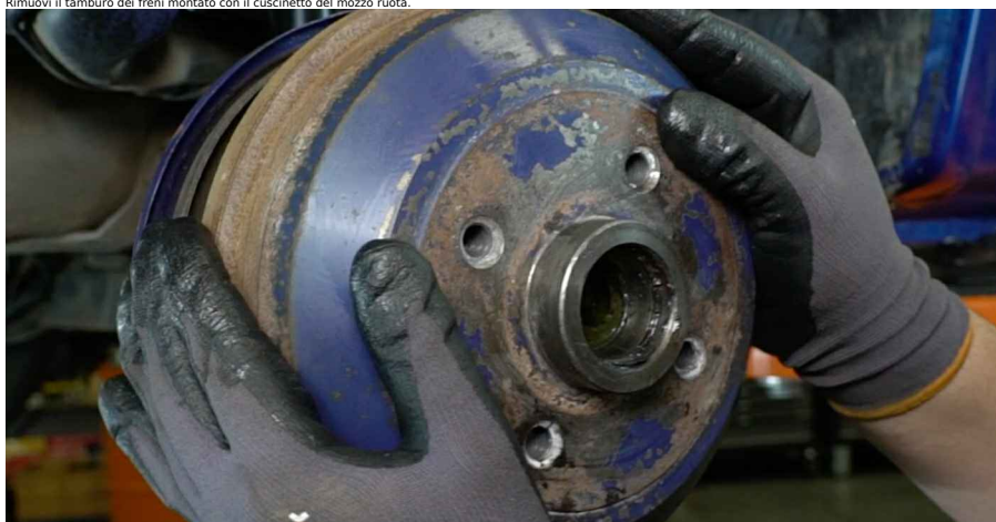
Sostituzione: cuscinetto ruota - VAUXHALL CORSAVAN Mk I (B). Il consiglio di AUTODOC:
