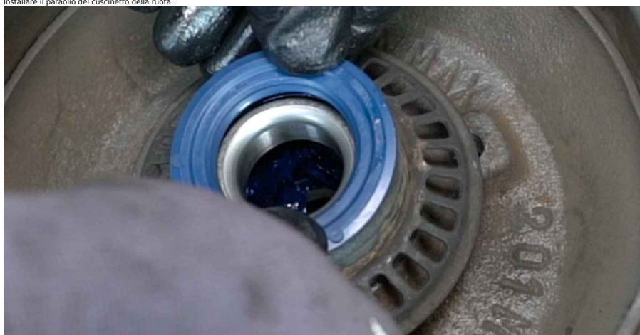
23 Applicare un prodotto trattante sul fusello. Usa un detergente spray multiuso. Utilizzare grasso per cuscinetti.
